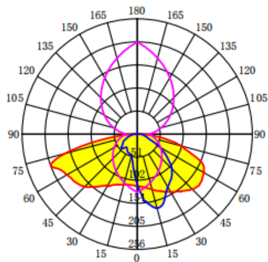
配光曲线
