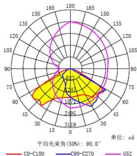
配光曲线
