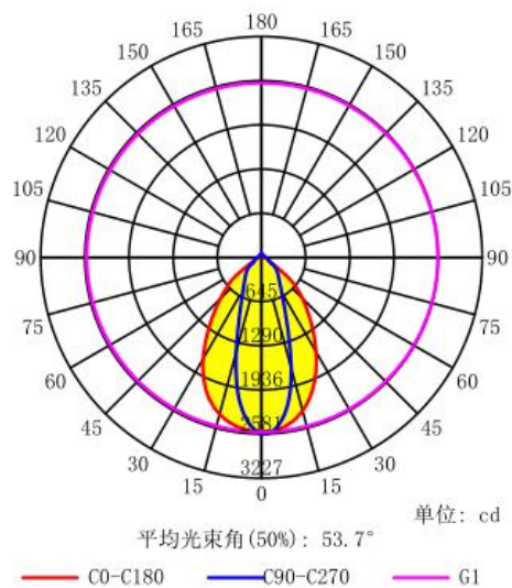
配光曲线
