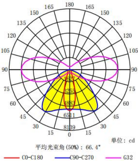
配光曲线
