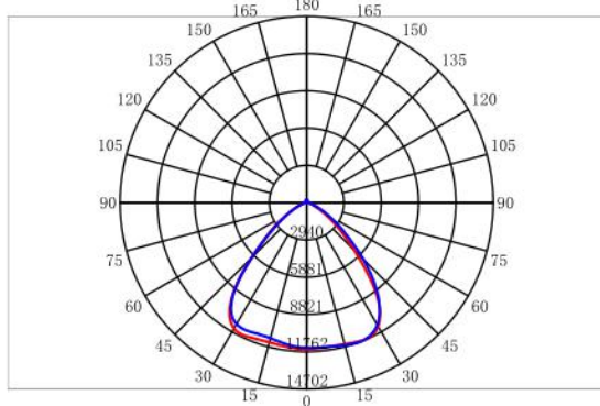
配光曲线
