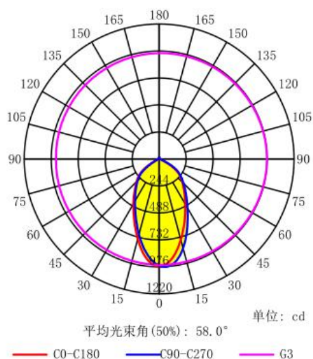
配光曲线
