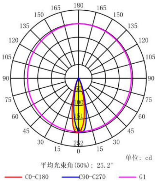
配光曲线
