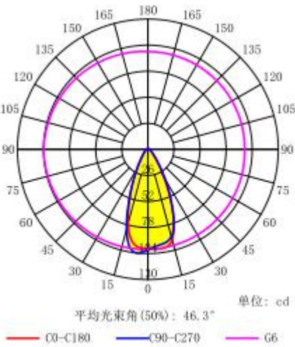
配光曲线
