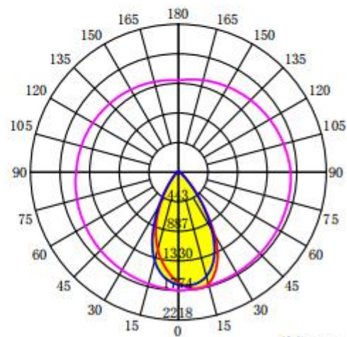
配光曲线
