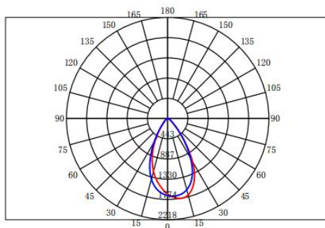
配光曲线
