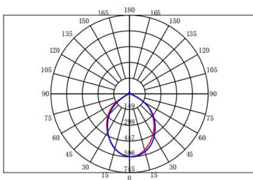
配光曲线
