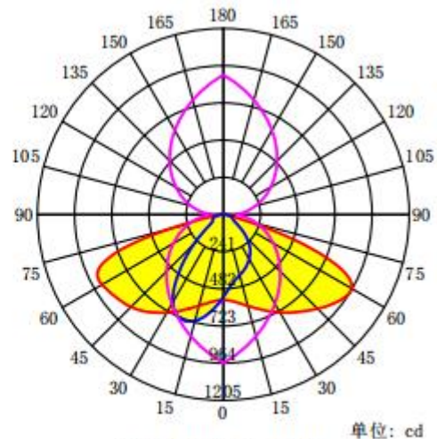
配光曲线
