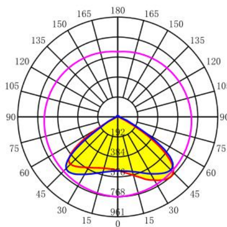
配光曲线
