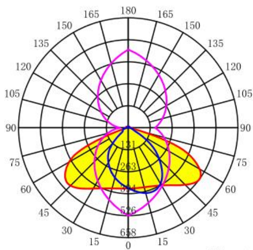
配光曲线
