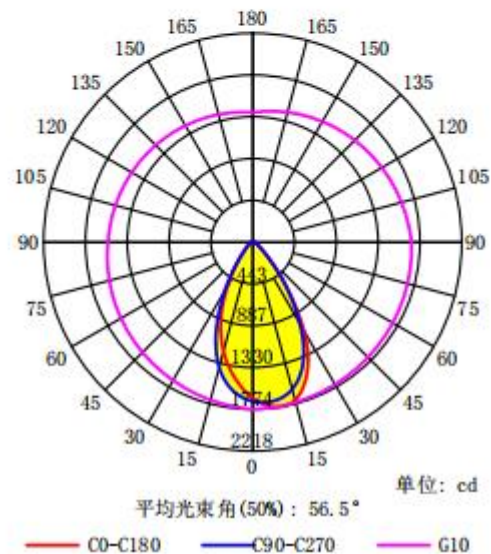
配光曲线
