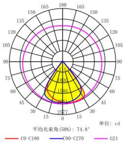
配光曲线
