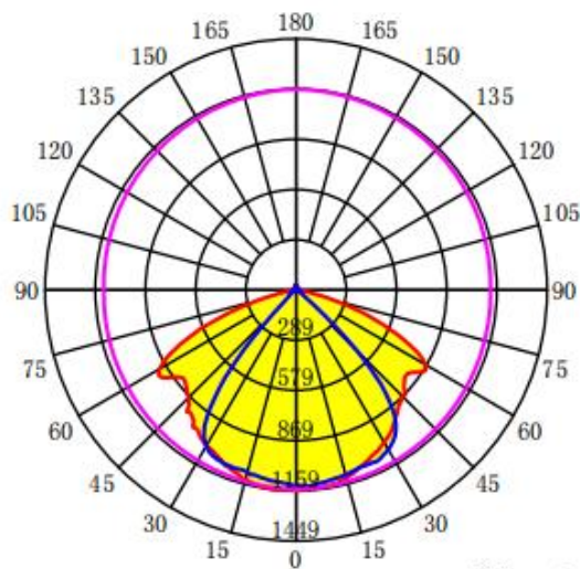
配光曲线
