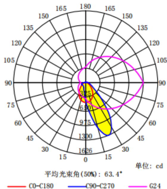
配光曲线
