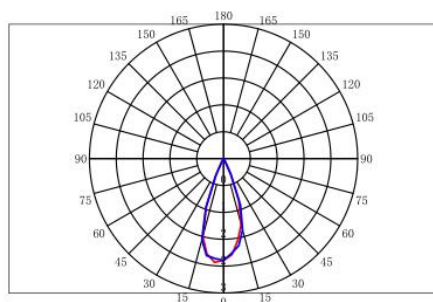
配光曲线
