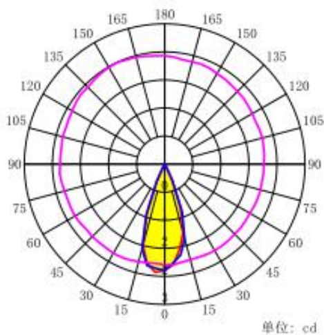
配光曲线
