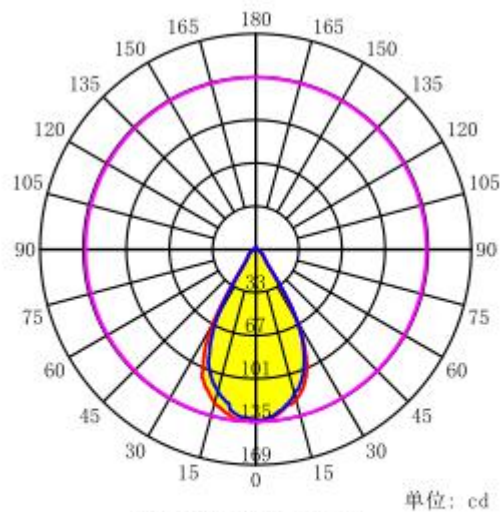
配光曲线
