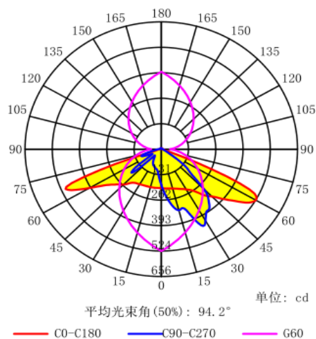
配光曲线
