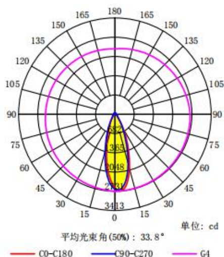
配光曲线
