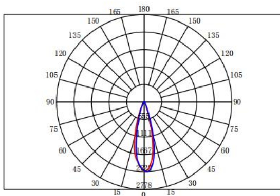
配光曲线
