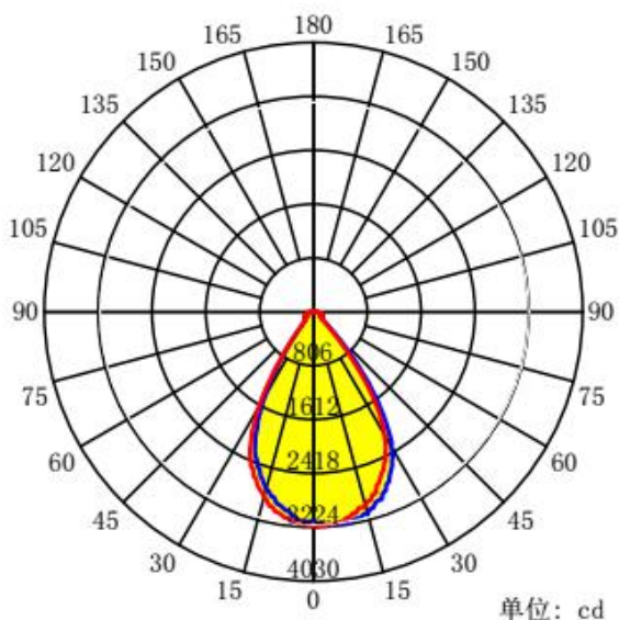
配光曲线
