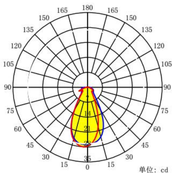
配光曲线
