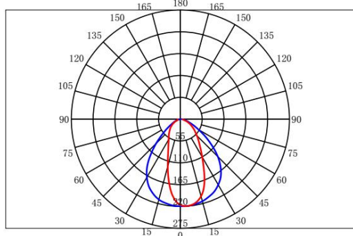
配光曲线
