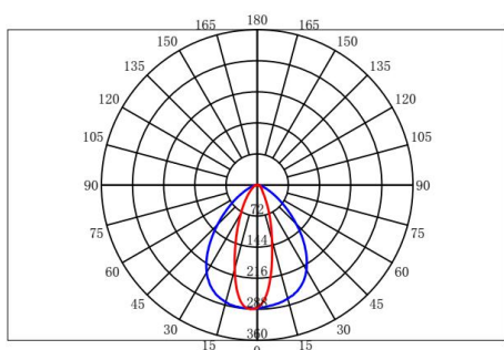
配光曲线
