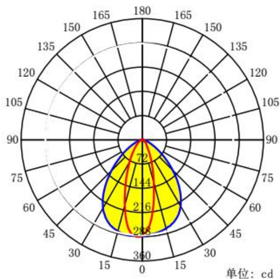
配光曲线
