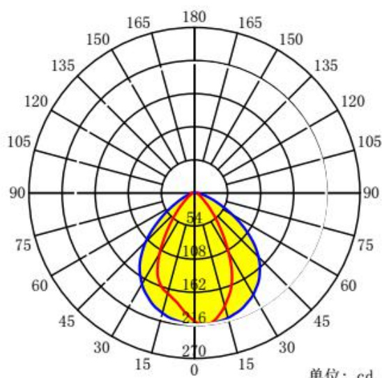
配光曲线
