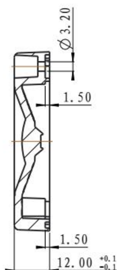
截面 AA-AA
