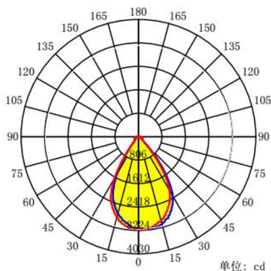
配光曲线
