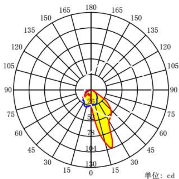
配光曲线
