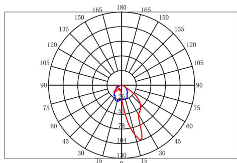
配光曲线
