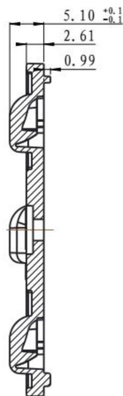
截面 A-A
