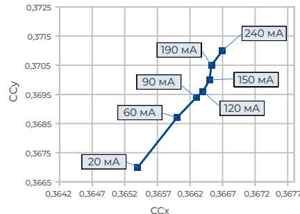
Типичная зависимость световых координат от прямого тока (Tj = 25 °C)
