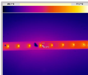
Термограмма, модуль NEO-L-45LS2835 ток 750 мА, T_a = 25^\circ\text{C} , установившийся тепловой режим, радиатор-корпус светильника «Армстронг»
