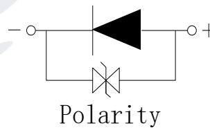
Fig.1-4 Polarity 极性
