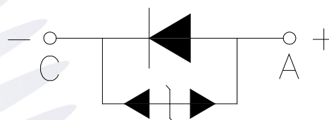
Fig.1-4 Polarity 极性
