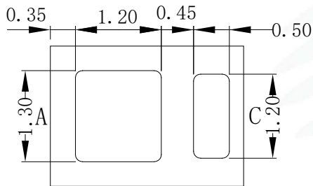
Fig.1-3 Bottom View 背面视图
