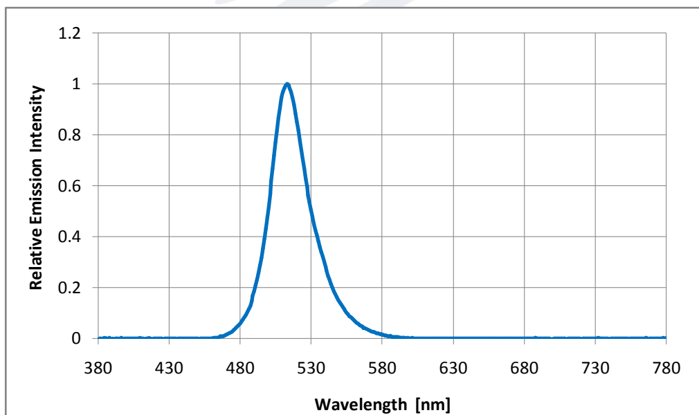
Fig 1-12 Spectrum Distribution 光谱分布特性曲线
