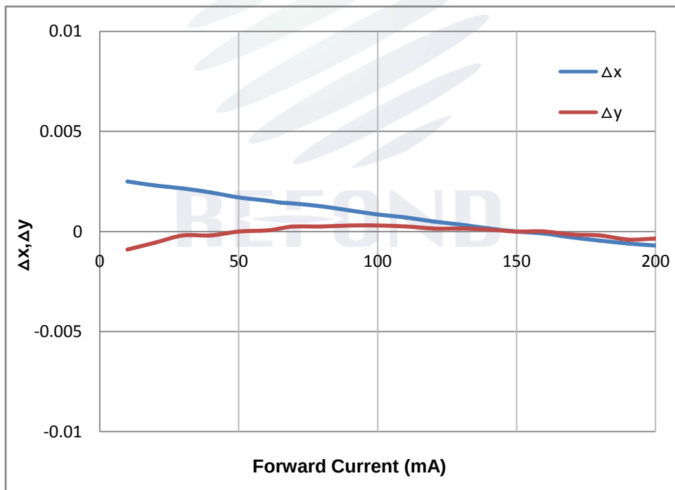
Fig 1-14 \Delta CIE_x, CIE_y vs Forward Current xy与电流特性曲线
