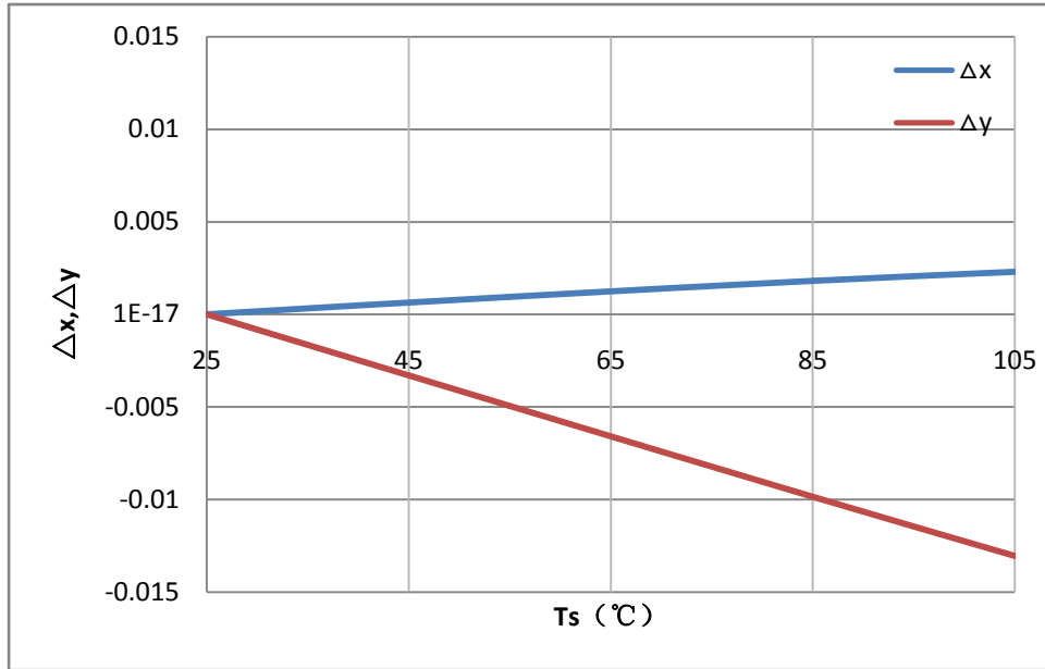
Fig 1-13 \Delta CIE_x, CIE_y vs Temperature xy与温度特性曲线
