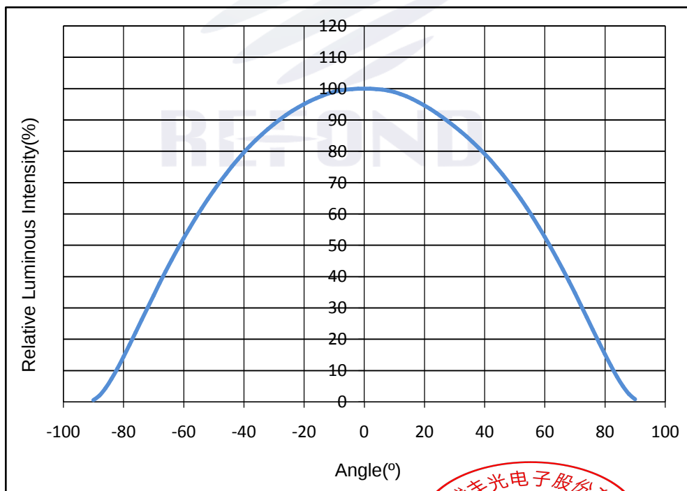
Fig 1-14 Radiation diagram 辐射特性曲线
