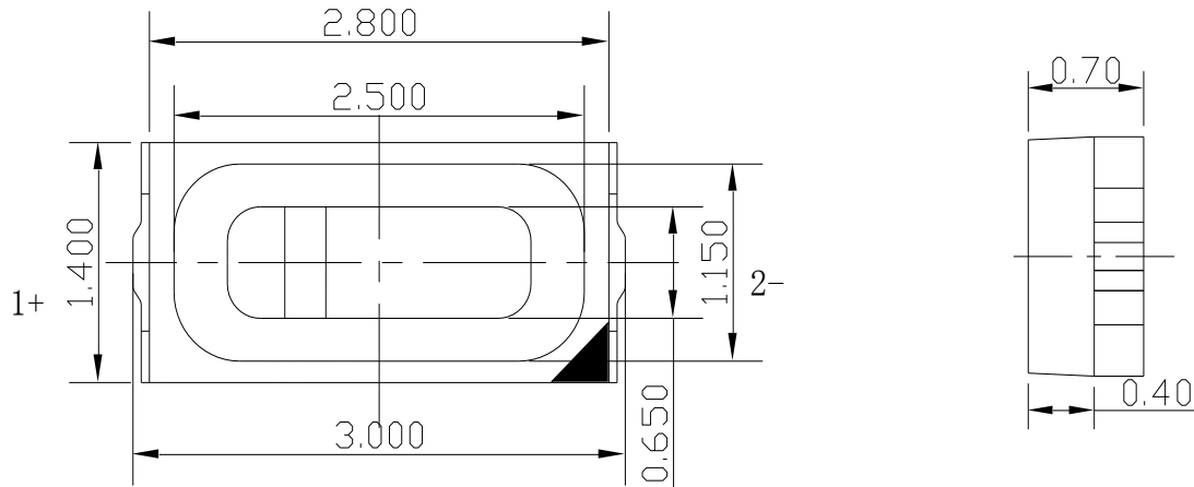
Fig.1-1 Top view 正面视图 Fig.1-2 Side view 侧面视图
