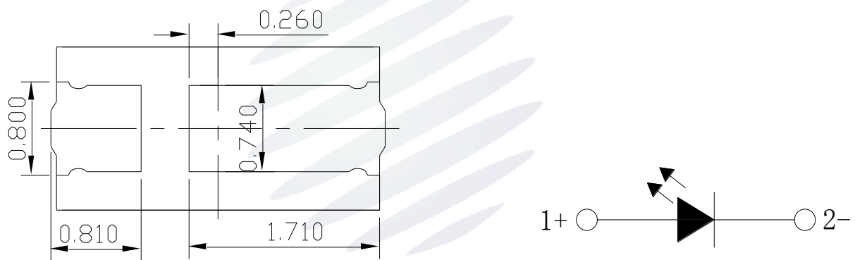
Fig.1-3 Bottom view 背面视图 Fig.1-4 Polarity 极性
