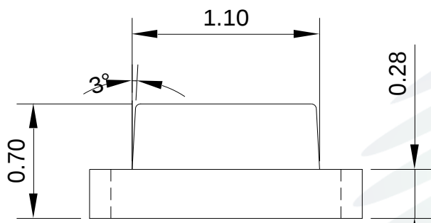
Fig.1-3 Bottom view 侧面视图
