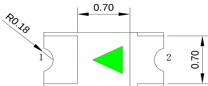
Fig.1-2 Side view 背面视图
