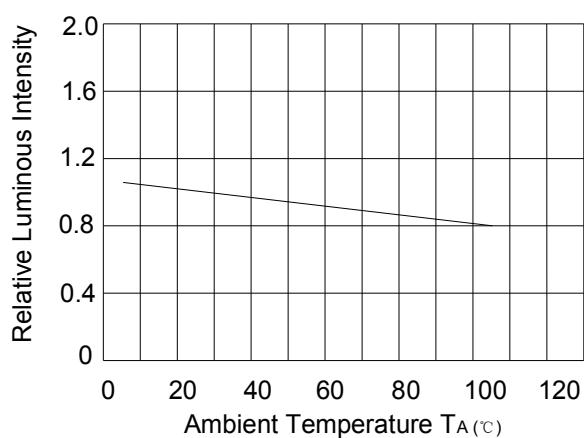
Fig.4 相对亮度 Vs. 环境温度
