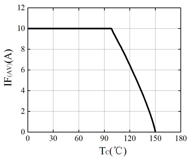
I_F vs T_C
