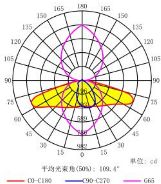
配光曲线
