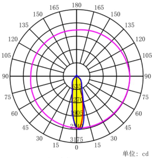
配光曲线
