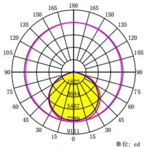
配光曲线
