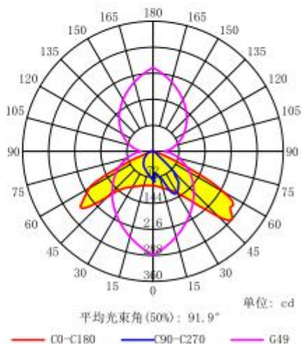
配光曲线
