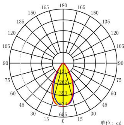
配光曲线
