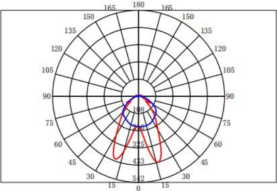
配光曲线
