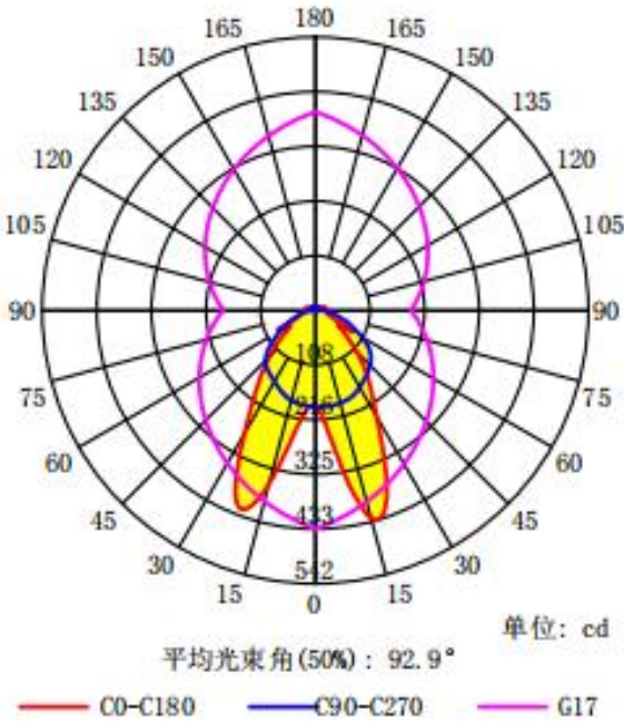
配光曲线
