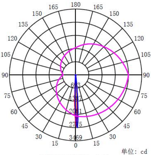
配光曲线
