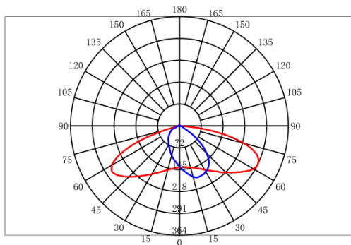
配光曲线
